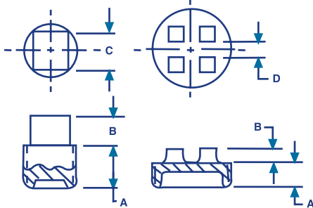
CABEZA CON RANURAS
